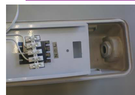
5-polige Anschlussklemme
