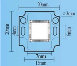
10W-20W Single-Chip / Einzelchip
