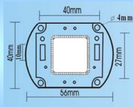
30W-200W Single-Chip / Einzelchip
